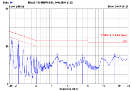
CISPR22 CLASS B AV 230V/50Hz 100% LOAD MARGIN: >7 dB
