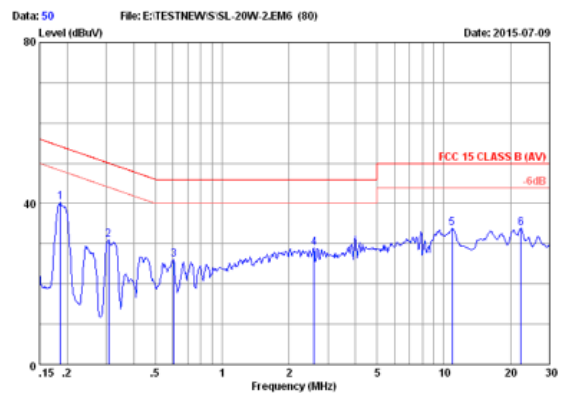
FCC15 CLASS B AV 100V/60Hz 100% LOAD MARGIN: >13 dB
