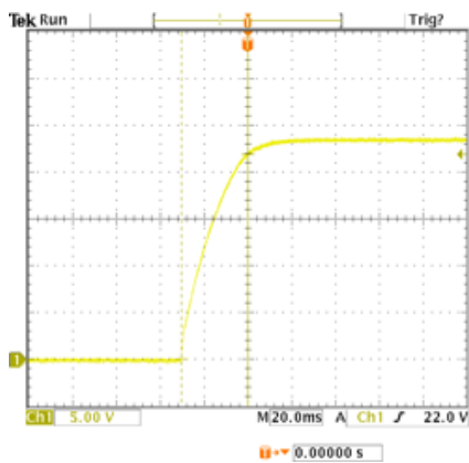
24V Rise Time
