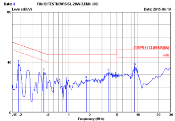
CISPR22 CLASS B AV 230V/50Hz 100% LOAD MARGIN: >14 dB
