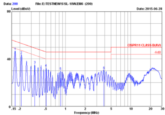
CISPR22 CLASS B AV 230V/50Hz 100% LOAD MARGIN: >08 dB
