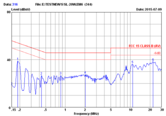
FCC15 CLASS B AV 100V/60Hz 100% LOAD MARGIN: >11 dB
