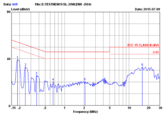
FCC15 CLASS B AV 100V/60Hz 100% LOAD MARGIN: >14 dB
