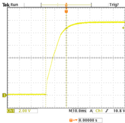
12V Rise Time
