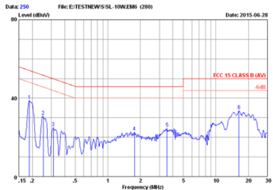
FCC15 CLASS B AV 100V/60Hz 100% LOAD MARGIN: >15 dB
