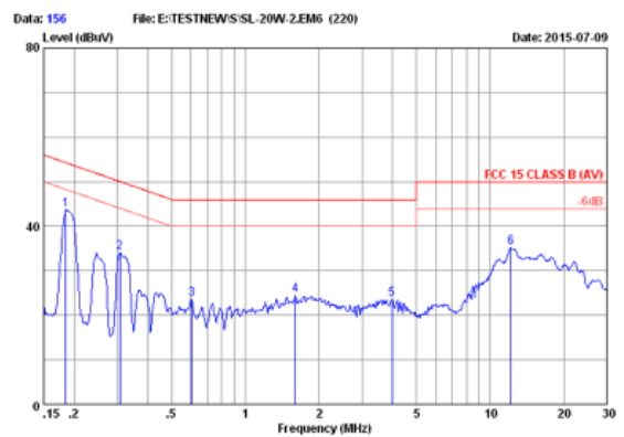
FCC15 CLASS B AV 100V/60Hz 100% LOAD MARGIN: >10 dB
