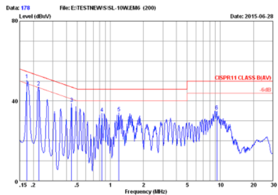
CISPR22 CLASS B AV 230V/50Hz 100% LOAD MARGIN: >4 dB
