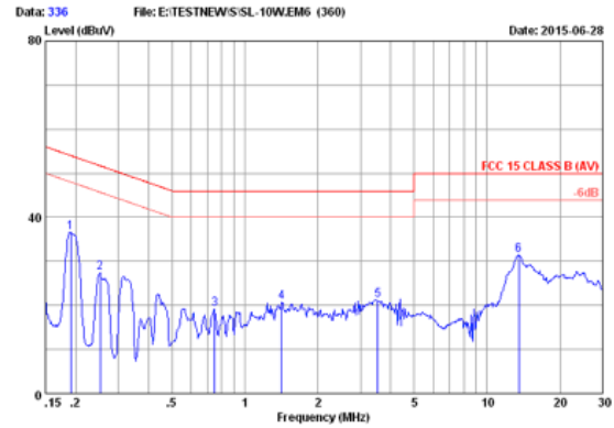
FCC15 CLASS B AV 100V/60Hz 100% LOAD MARGIN: >17 dB
